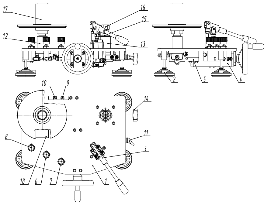
Рисунок 2. УСД НД с ИПС для диапазона 0,2...10.
