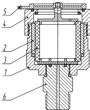
Рисунок 7. Устройство ИПС диапазона 0,2...0,5.
