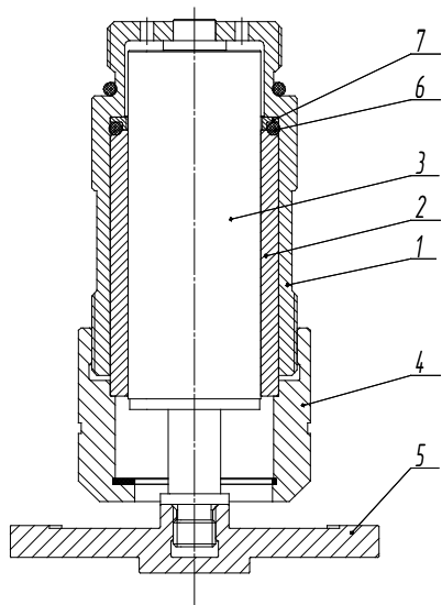
Рисунок 6. Устройство ИПС диапазона -1...0.
