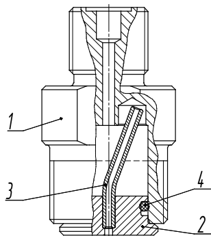
Рисунок 9. Устройство переходника-грязеуловителя.
