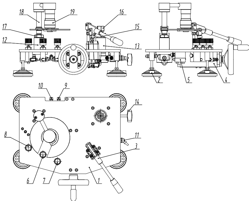
Рисунок 1. УСД НД с ИПС для диапазона -1...0.
