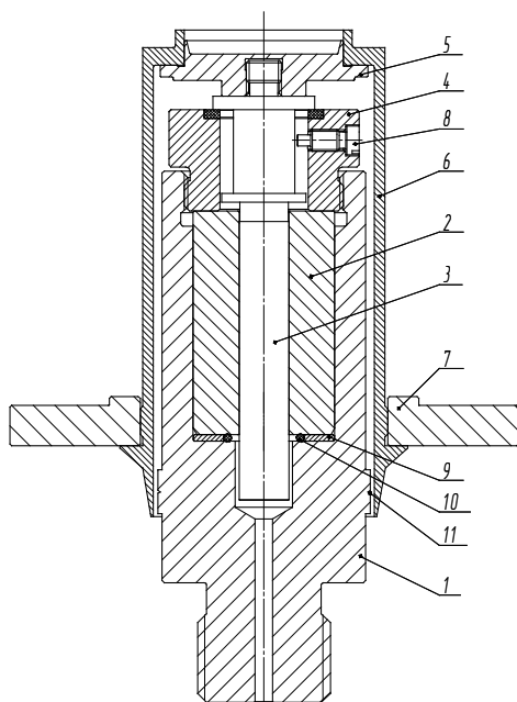
Рисунок 8. Устройство ИПС диапазона 1...160.
