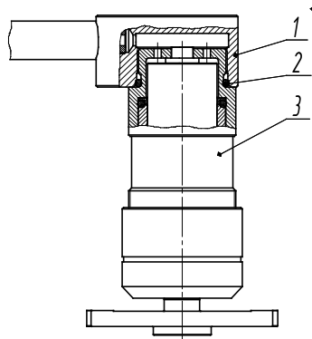
Рисунок 11. Установка ИПС на кронштейн МГП-В.
