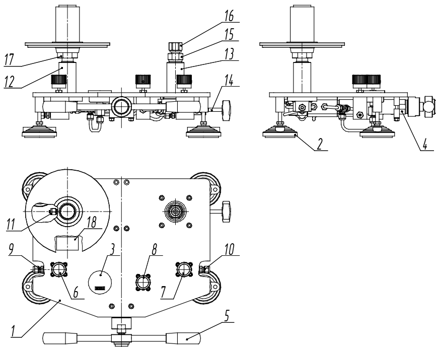
Рисунок 4. УСД ВД с ИПС для диапазона 1...160.
