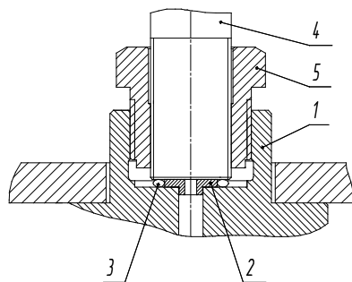
Рисунок 10. Установка кронштейна для МПП-В.
