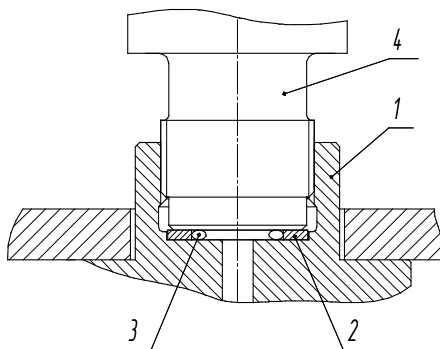
Рисунок 12. Установка ИПС на стойку МГП-0,2...МГП-160.
