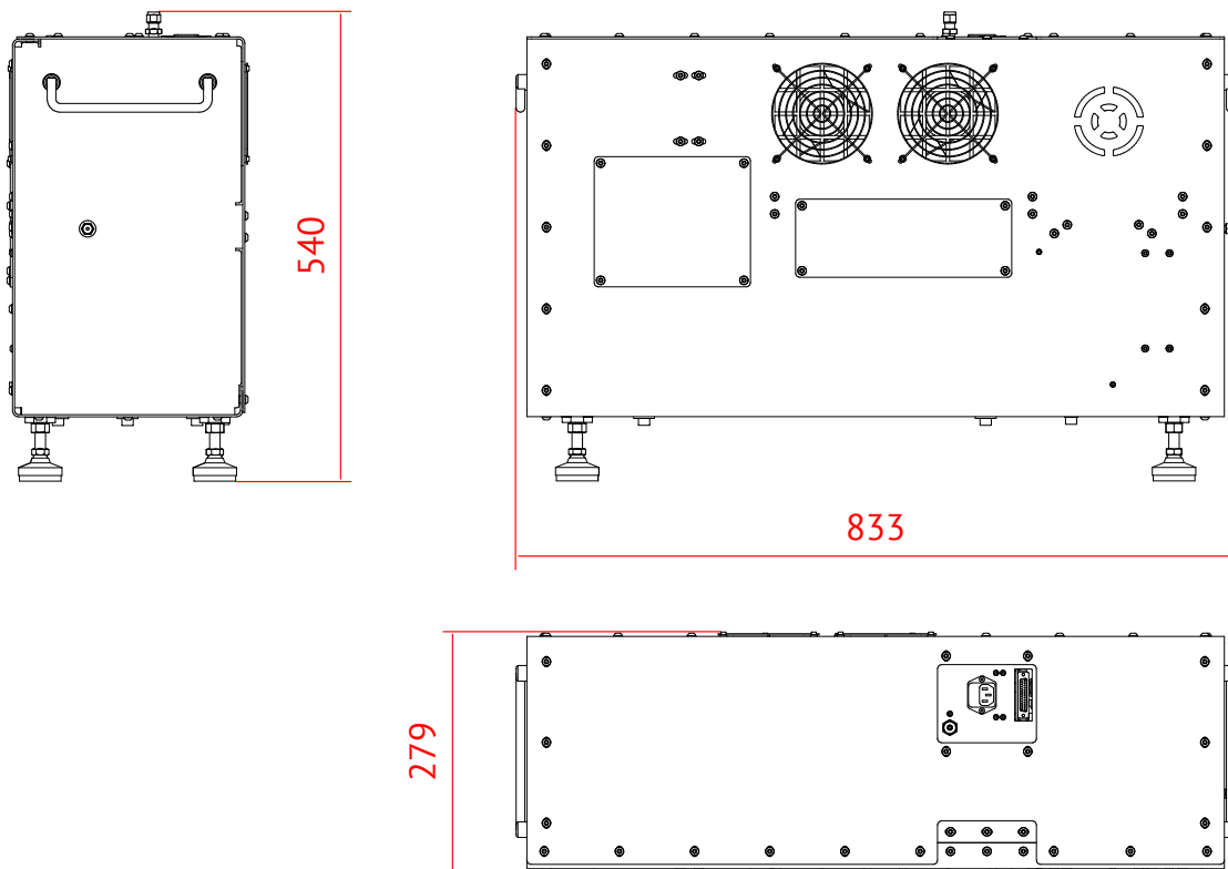
Рис. 2. Силовой блок.
