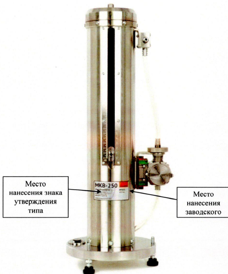
Рисунок 1 – Общий вид микроманометра МКВ-250
